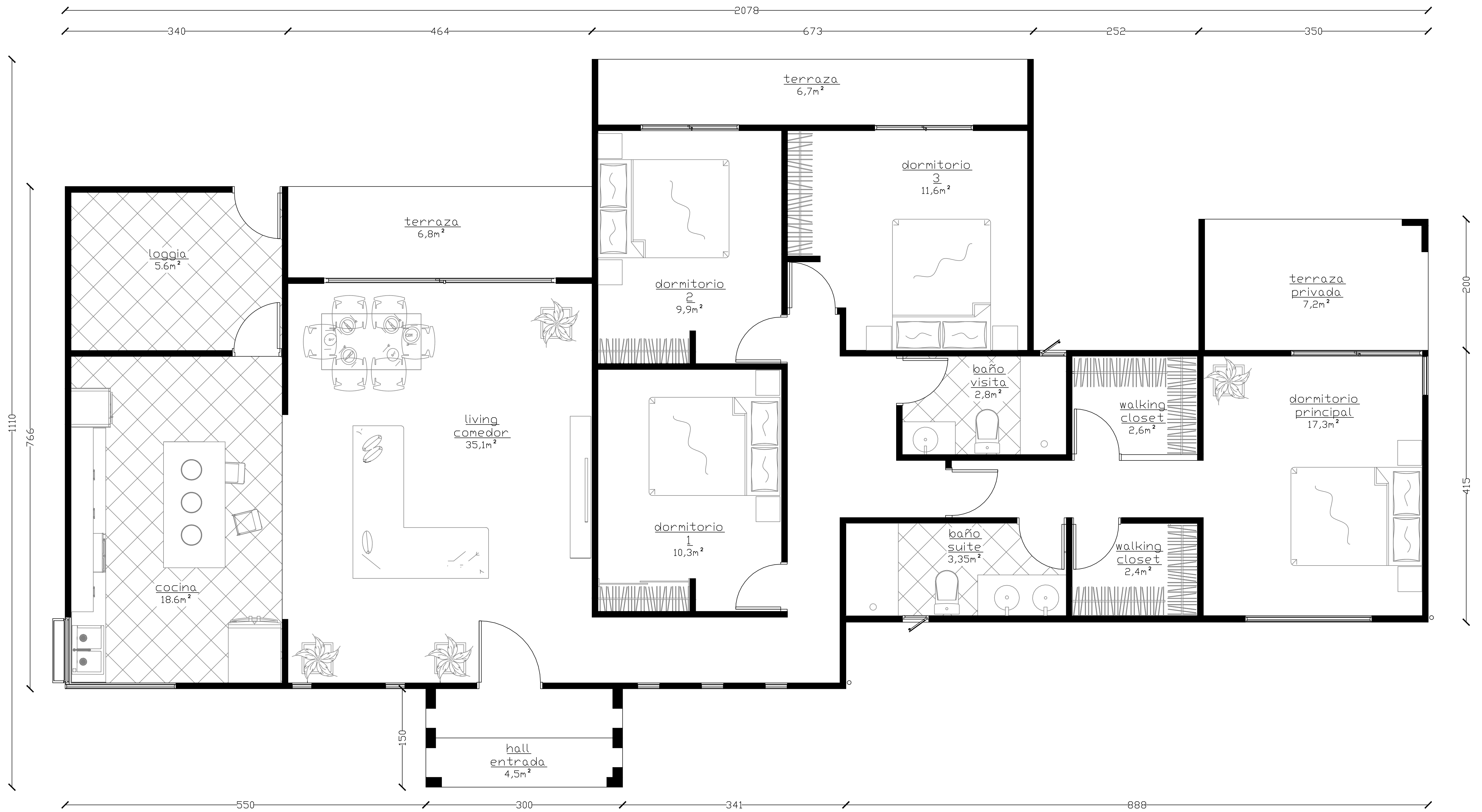
PLANO PLANTA ARQUITECTURA ESC 1:50 160m2
