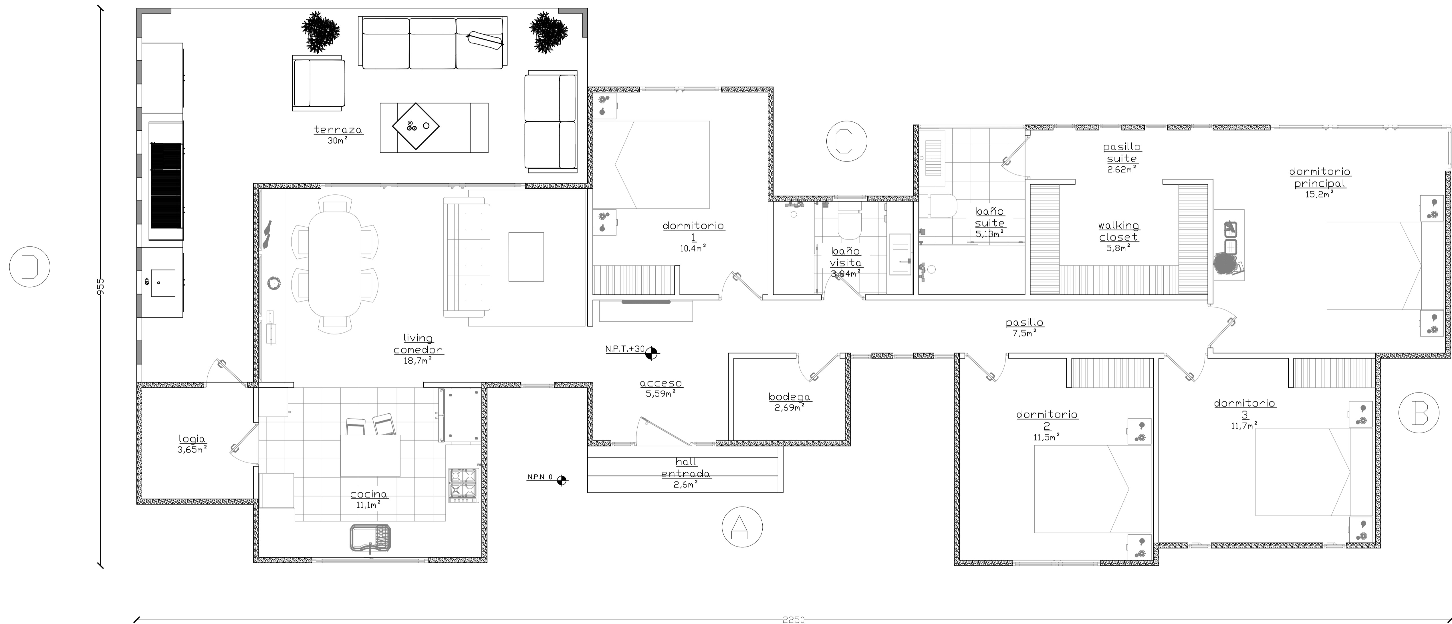
PLANO PLANTA ARQUITECTURA ESC 1:50 160m2
