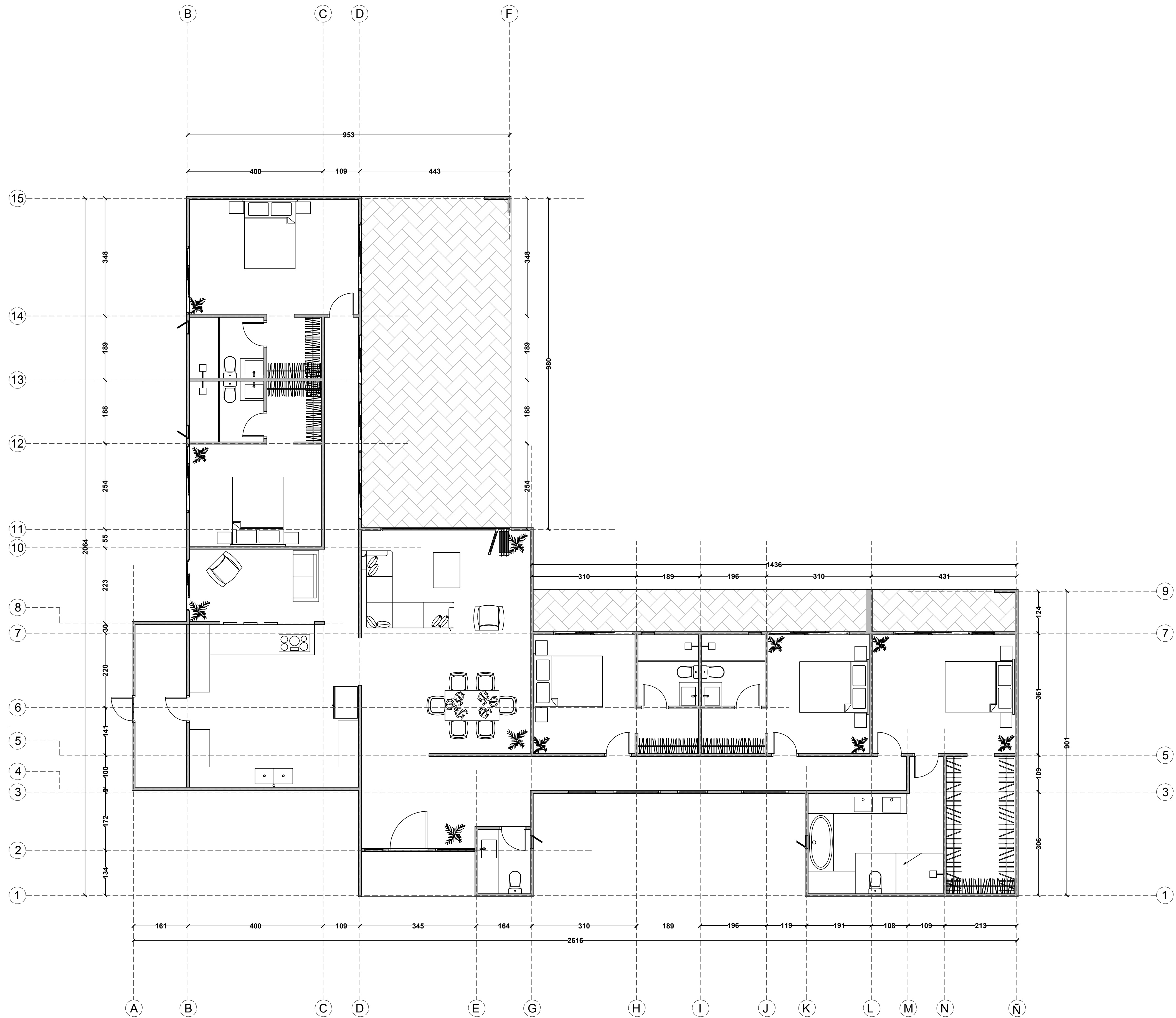
PLANTA ARQUITECTURA EJES ESC 1:50
