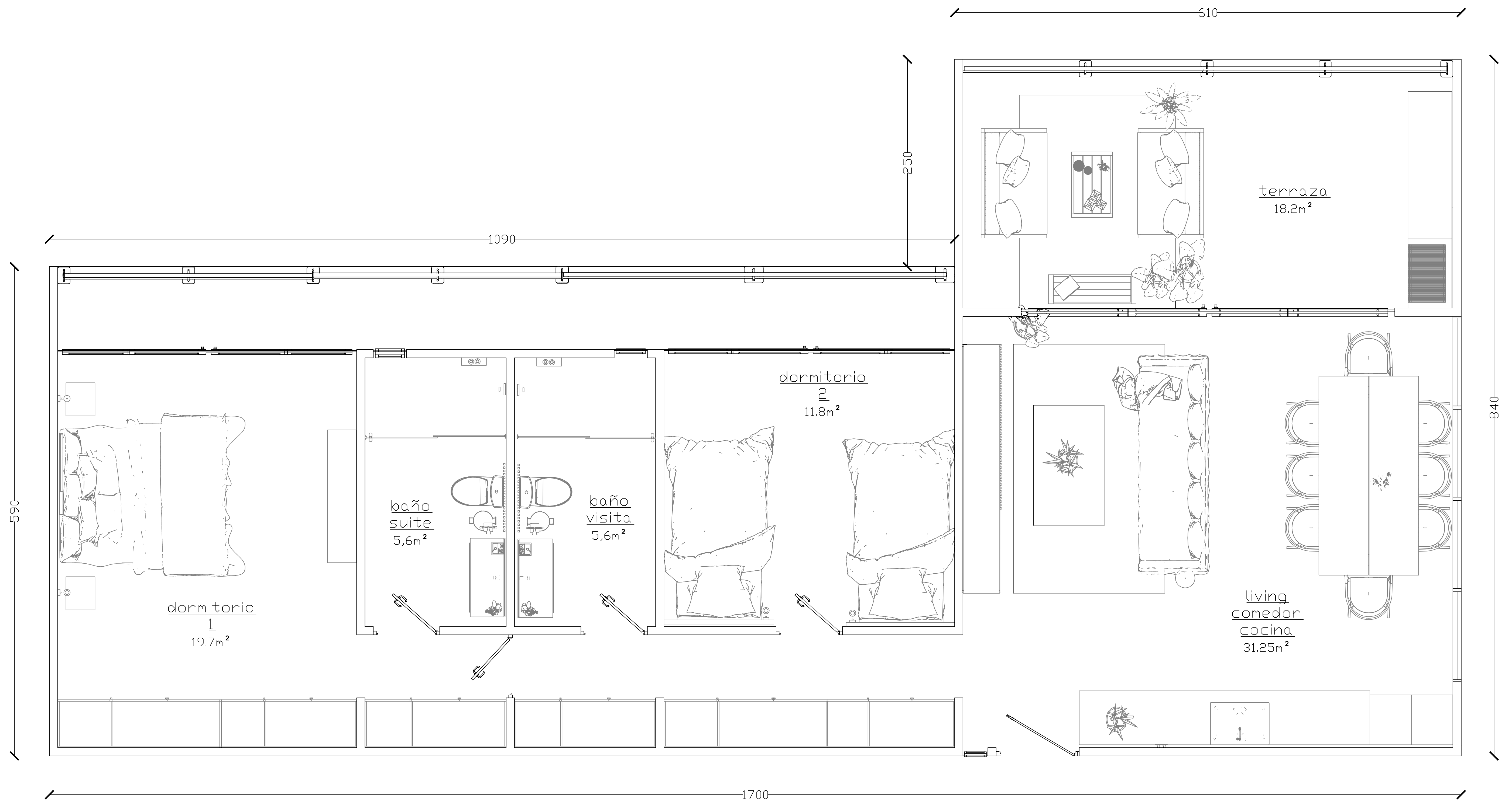
PLANO PLANTA ARQUITECTURA ESC 1:50 116m 2
